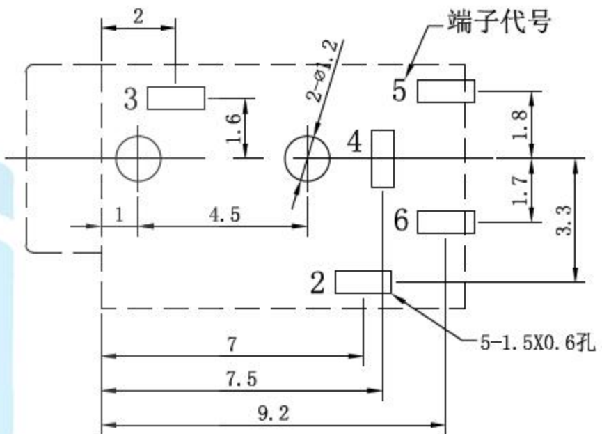
PCB. 开孔尺寸图 Top View
