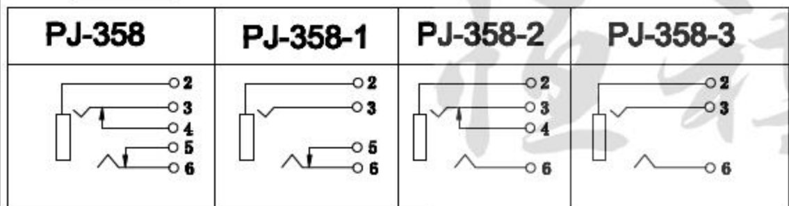
电路原理图
