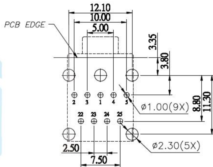
P.C.B LAYOUT
