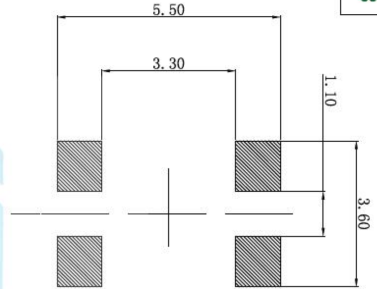
PCB. 焊接尺寸图
