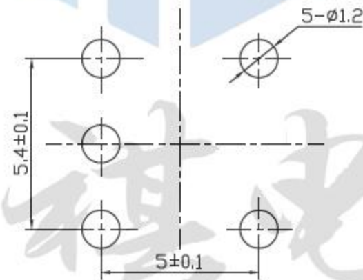
安装尺寸图
