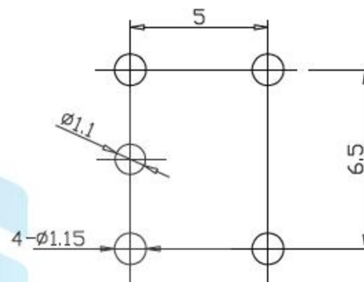
安装尺寸
