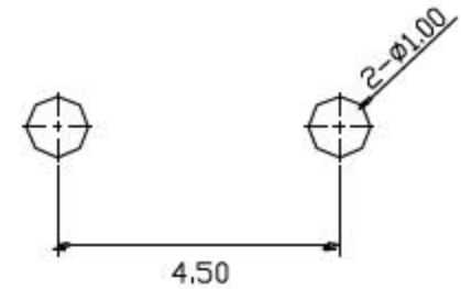
PCB. 焊接图
