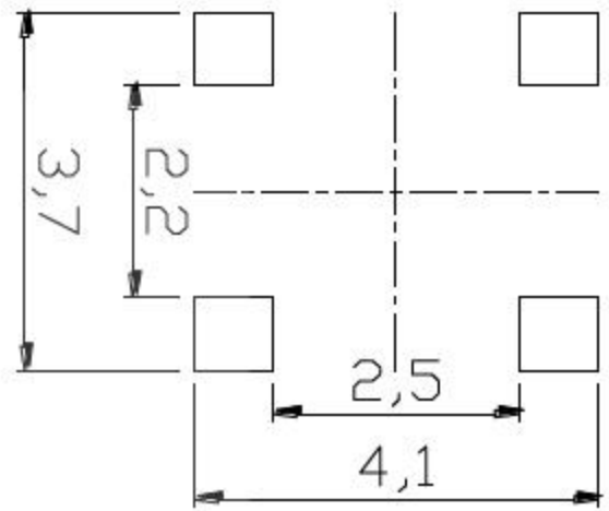
PCB. 焊接图
