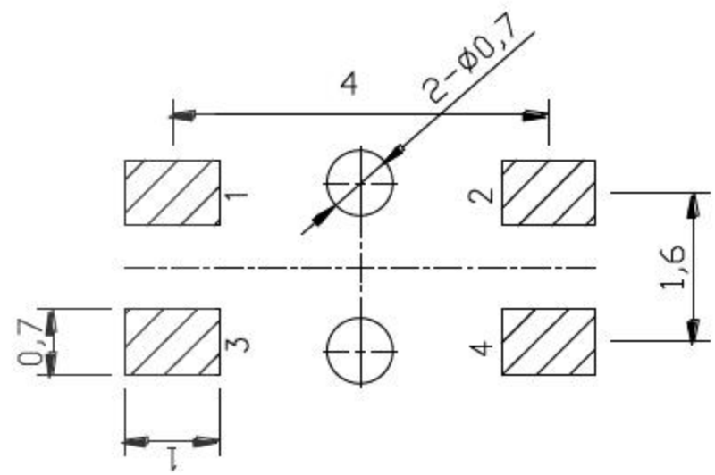
PCB. 焊接图
