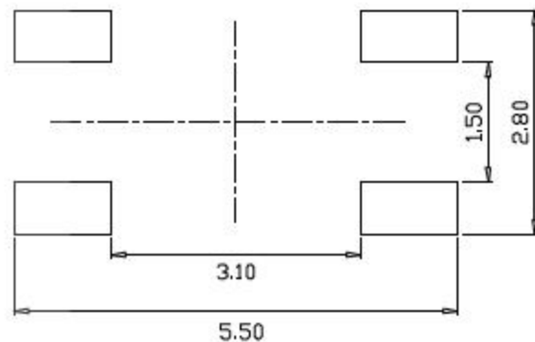
PCB. 焊接图
