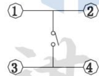
电路图
