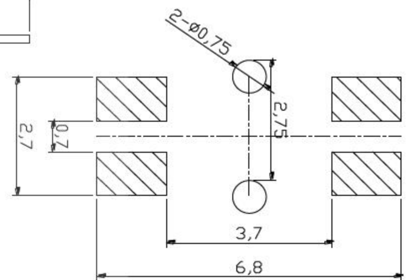
PCB. 焊接图
