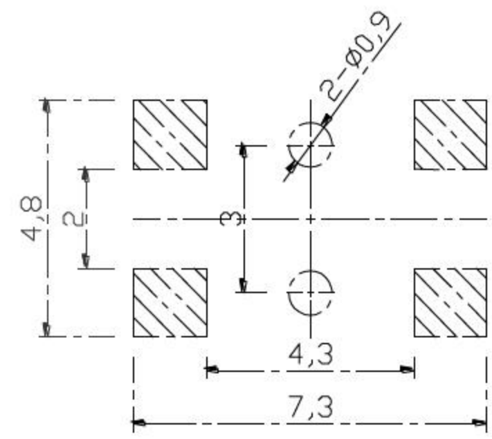
PCB. 焊接图
