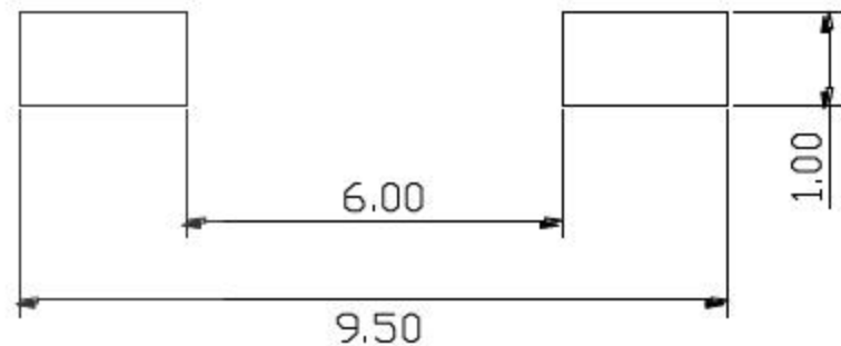
PCB. 焊接图
