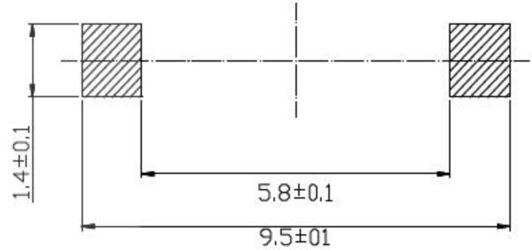
PCB. 焊接尺寸图
