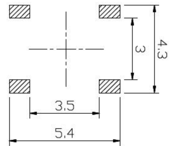
PCB. 焊接图
