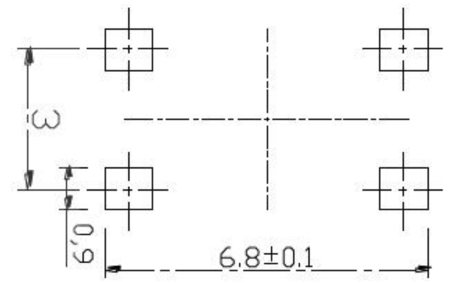
PCB. 焊接图
