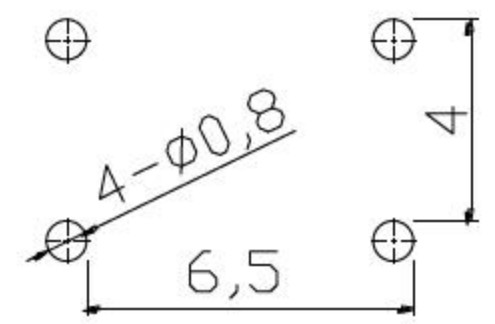
PCB. 焊接图
