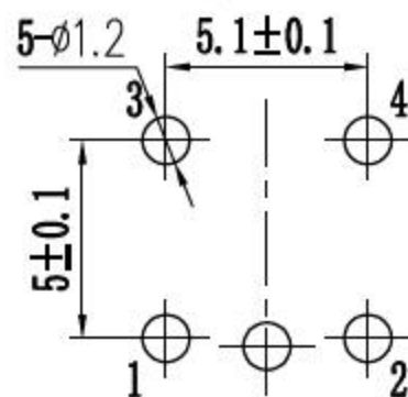
元件面孔位图
