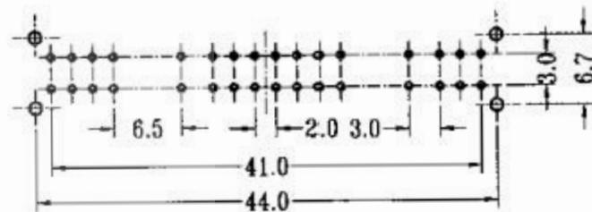
P.C.B LAYOUT
