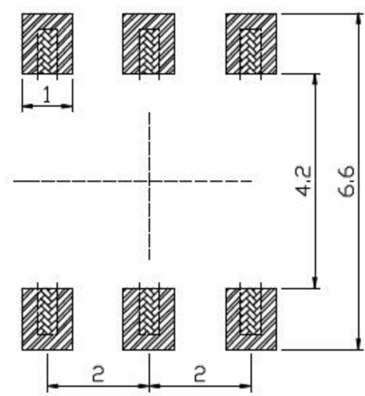
安装图 (PCB LAYOUT PLAN)
