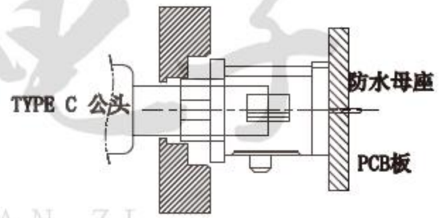
组装示意图
