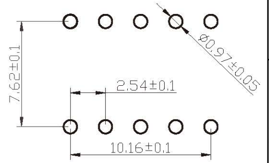
PCB开孔
