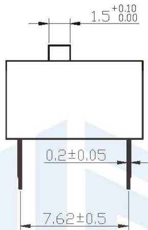
高推钮 (E)
