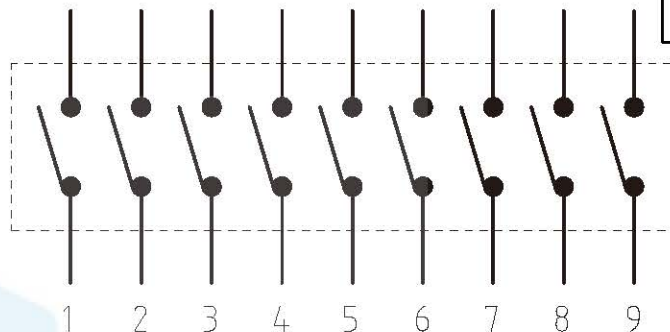
电路图
