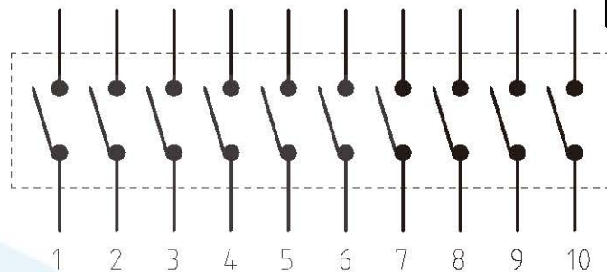
电路图
