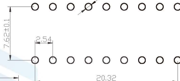
PCB开孔
